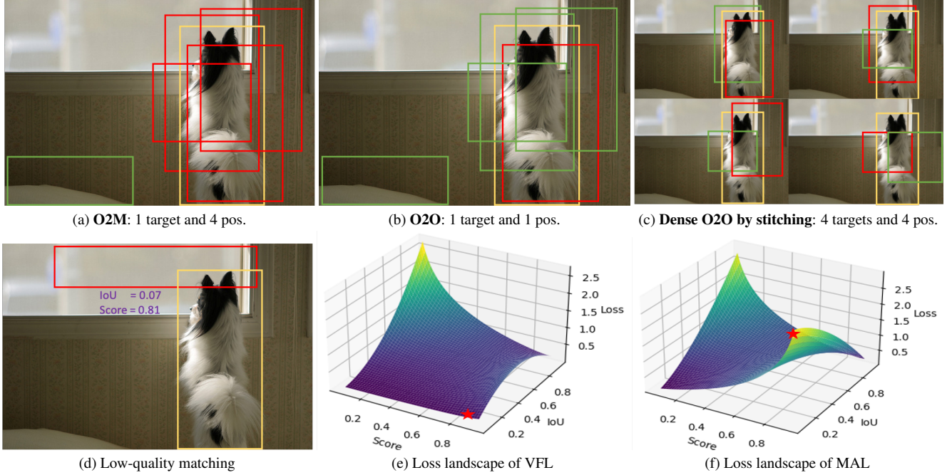
图2. 我们提出的DEIM示意图。黄色、红色和绿色框分别代表GT、正样本和负样本。"pos."表示正样本。 Top : 我们的密集O2O（图2c）能提供与O2M（图2a）同等质量的正样本。 Bottom : 对于低质量匹配，使用VFL[40]和MAL时的损失值分别标记为 \star ，表明MAL能更有效地优化这些情况。
